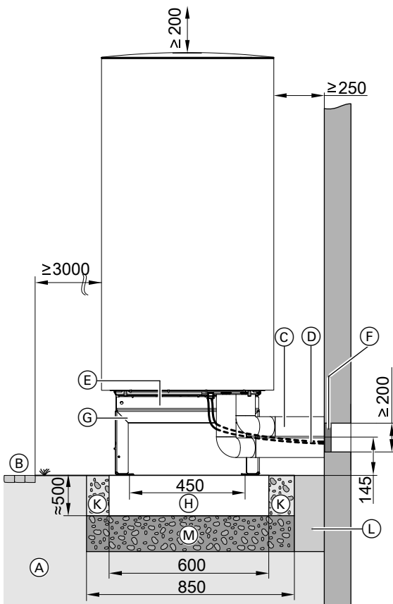
Afb. 25 Max. wandafstand met design-bekleding (accessoires): 300 mm
