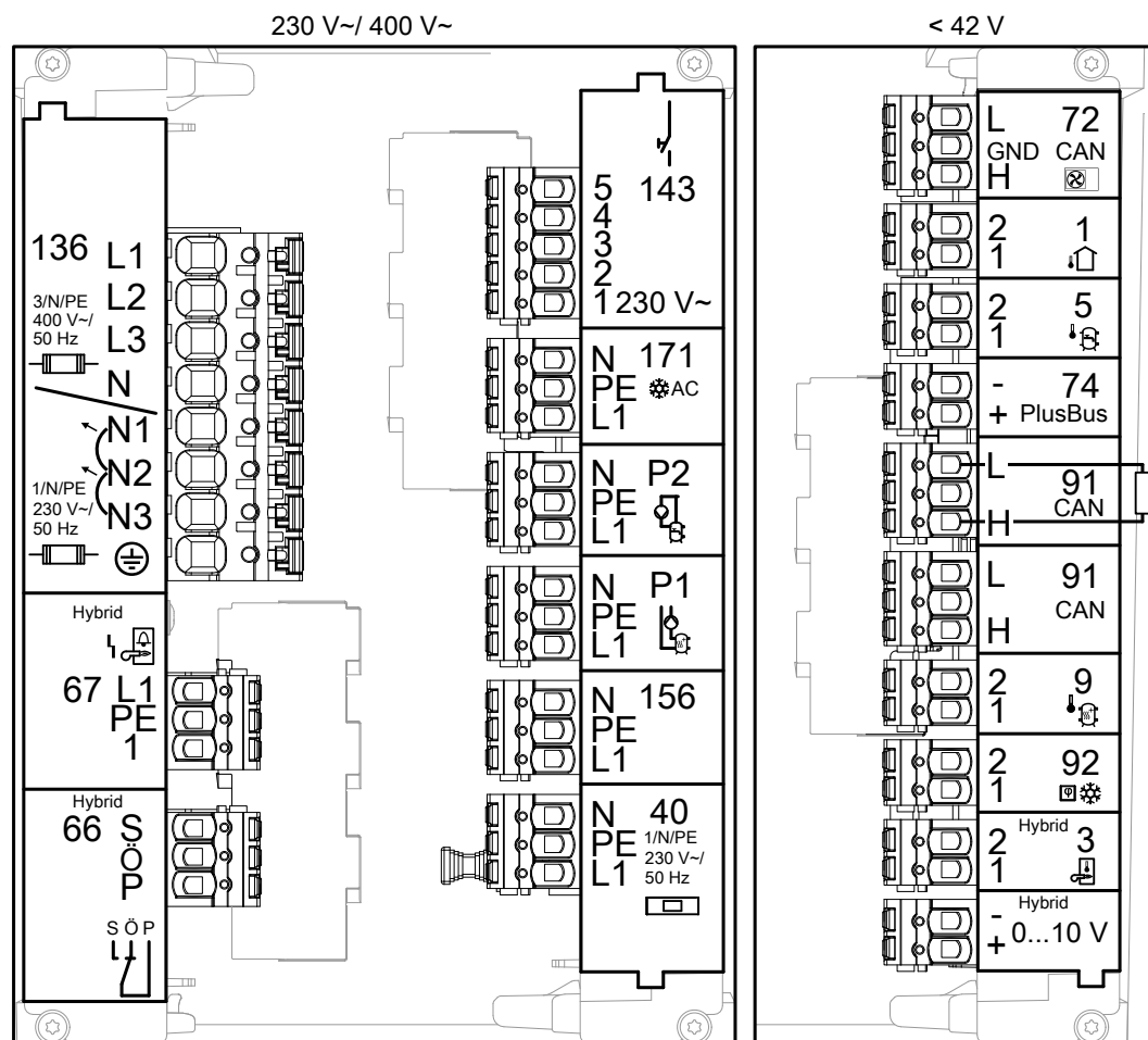
Afb. 41 Uitleg van de aansluitingen: zie volgende tabellen.
