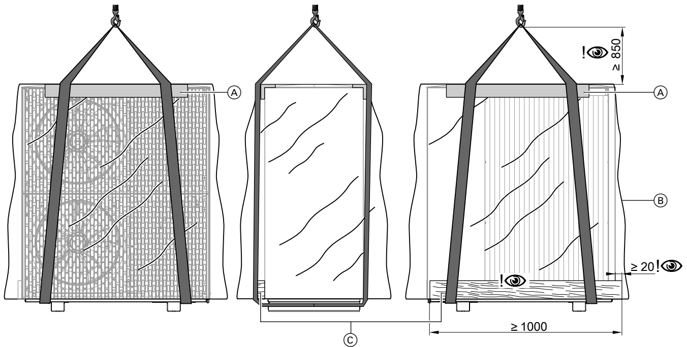
Afb. 8 Transport met kraan als voorbeeld van de buitenunit met 2 ventilatoren
